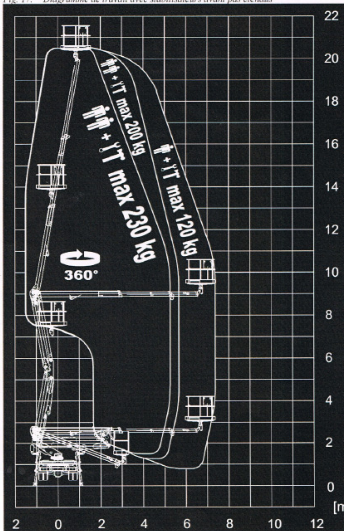
Fig. 17. Diagramme de travail avec stabilisateurs avant pas étendus
